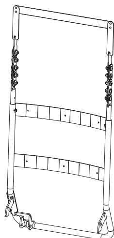
Rücken RG70 - mit Gliederkette - AL Anb. 175 mm Art-Nr. RG 70-015912
