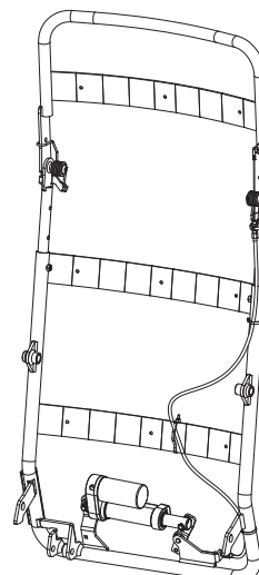
Rücken RG70 - Motorische Kopfstütze (30° KS) - AL Anb. 175 mm Art-Nr. RG 70-015693
