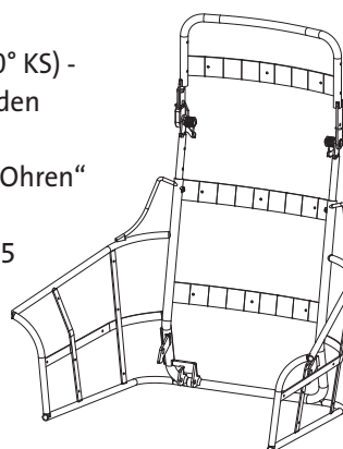
Rücken RG70 - Rastgelenk (30° KS) - mit umlaufenden Armlehnen - Optional mit „Ohren“ Art-Nr. RG 70-015920
